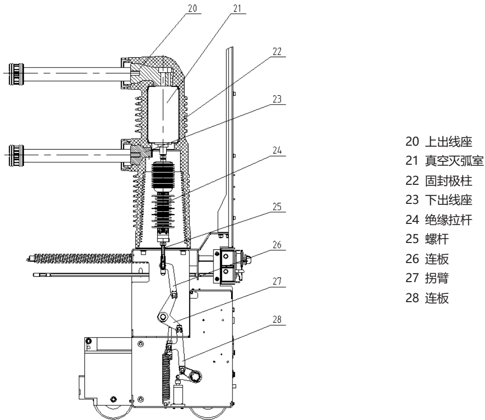
图 3 断路器内部结构图 (落地式)
