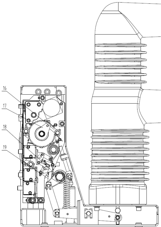
图2 断路器操动机构侧视
