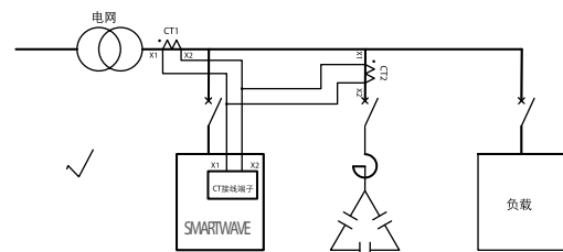
CT 接在电源侧，正确接法
