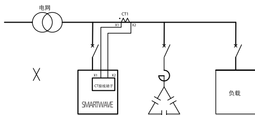
CT 接在负载侧，错误接法
