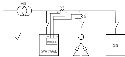
CT 接在负载侧，正确接法
