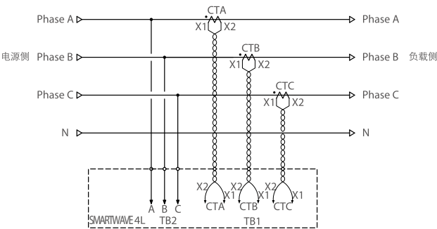
SMARTWAVE 4L 电流互感器接在负载侧的配线示意图
