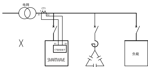
CT 接在电源侧，错误接法
