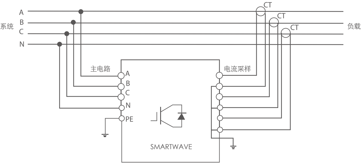
SMARTWAVE 三相四线制接线示意（用于商业建筑类负荷）
