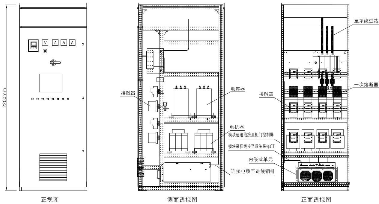
结构示意图
