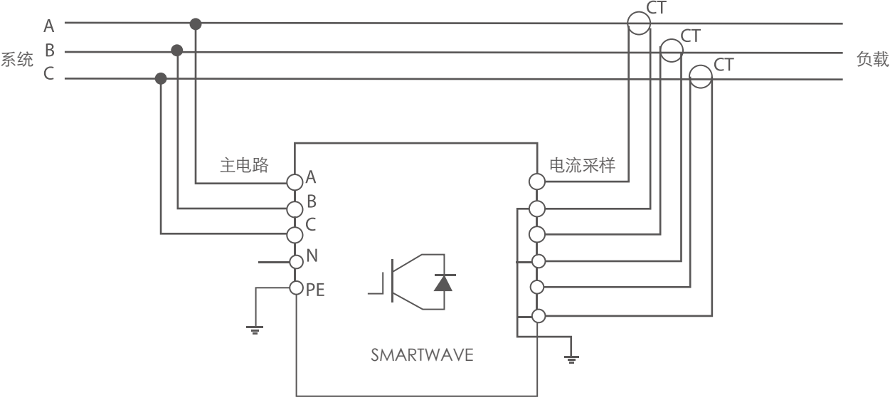
SMARTWAVE 三相三线制接线示意（用于工业类负荷）
