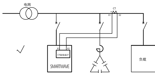
CT 接在负载侧，正确接法
