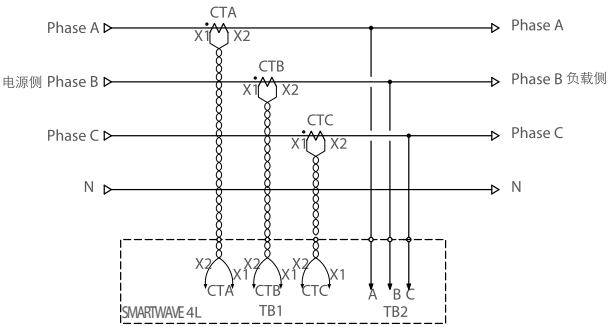
SMARTWAVE 4L 电流互感器接在电源侧的配线示意图
